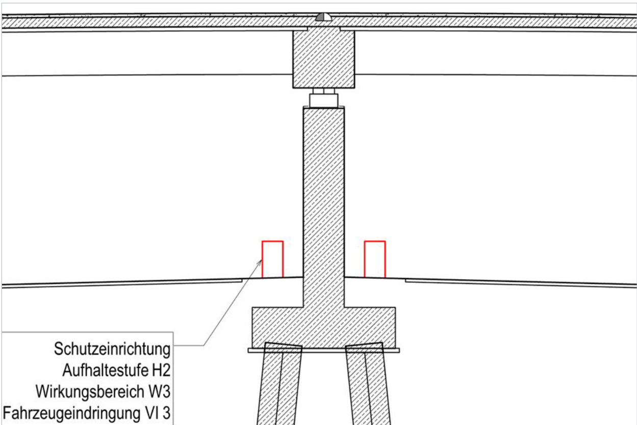
Abbildung 6: Schnitt durch vereinfachte Platzhalter von Schutzeinrichtungen inklusive textlicher Hinweise (Quelle: Schüßler-Plan digital)
