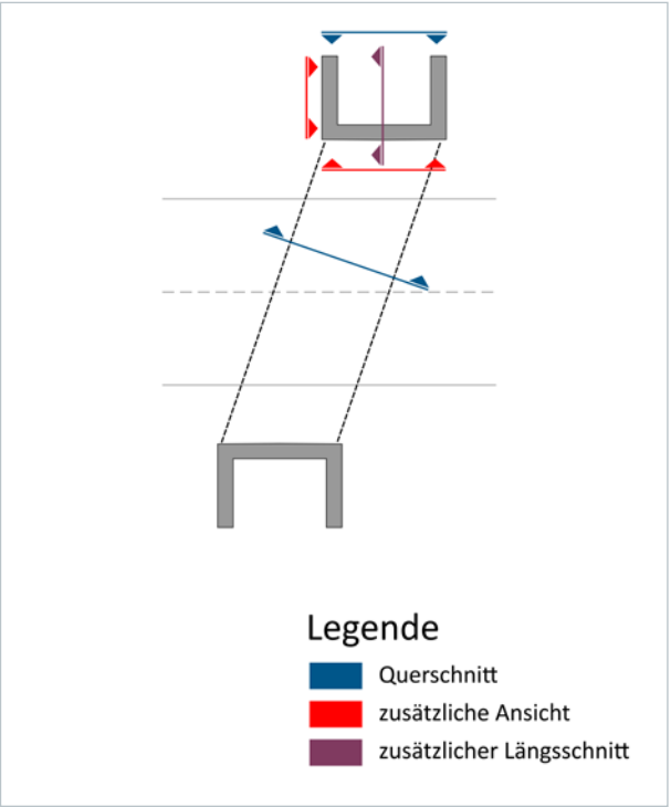
Abbildung 11: Beispiel 5 für mögliche Schnittführung und Ansichten für verschiedene Konstruktionsformen des Widerlagers (Quelle: Schüßler-Plan digital)
