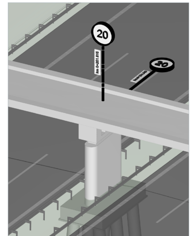
Abbildung 14: Raster eines Brückenbauwerks als 3D-Annotation (Quelle: Schüßler-Plan digital)
