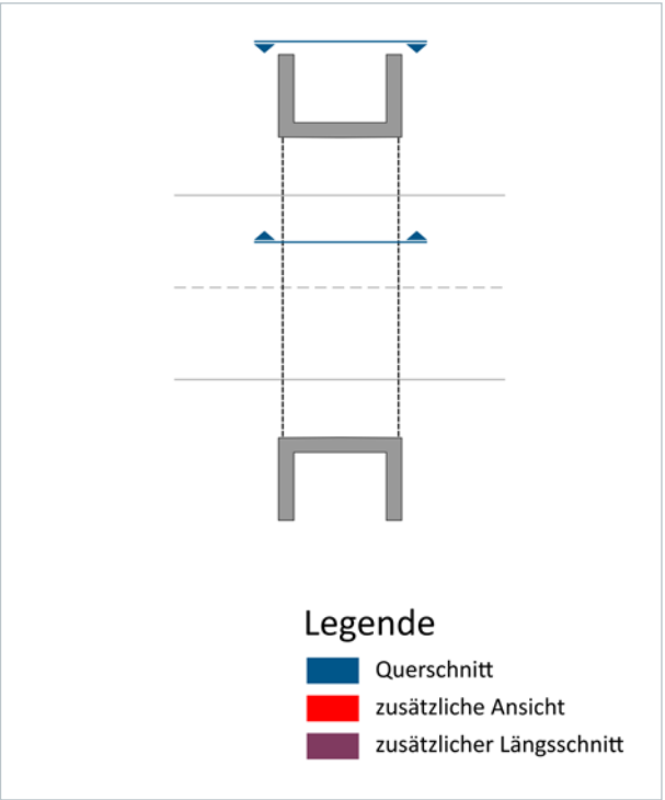
Abbildung 9: Beispiel 3 für mögliche Schnittführung und Ansichten für verschiedene Konstruktionsformen des Widerlagers (Quelle: Schüßler-Plan digital)
