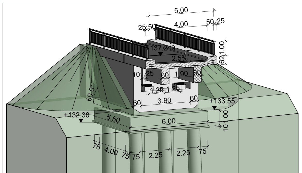
Abbildung 5: 3D-Ansicht mit orthogonalem Schnitt zur Bauwerksachse (© Schüler-Plan)
