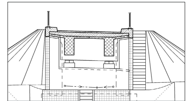
Abbildung 3: Geometrisch idealisierte Schnittdarstellung gemäß bestehender Konventionen (© Schüßler-Plan)
