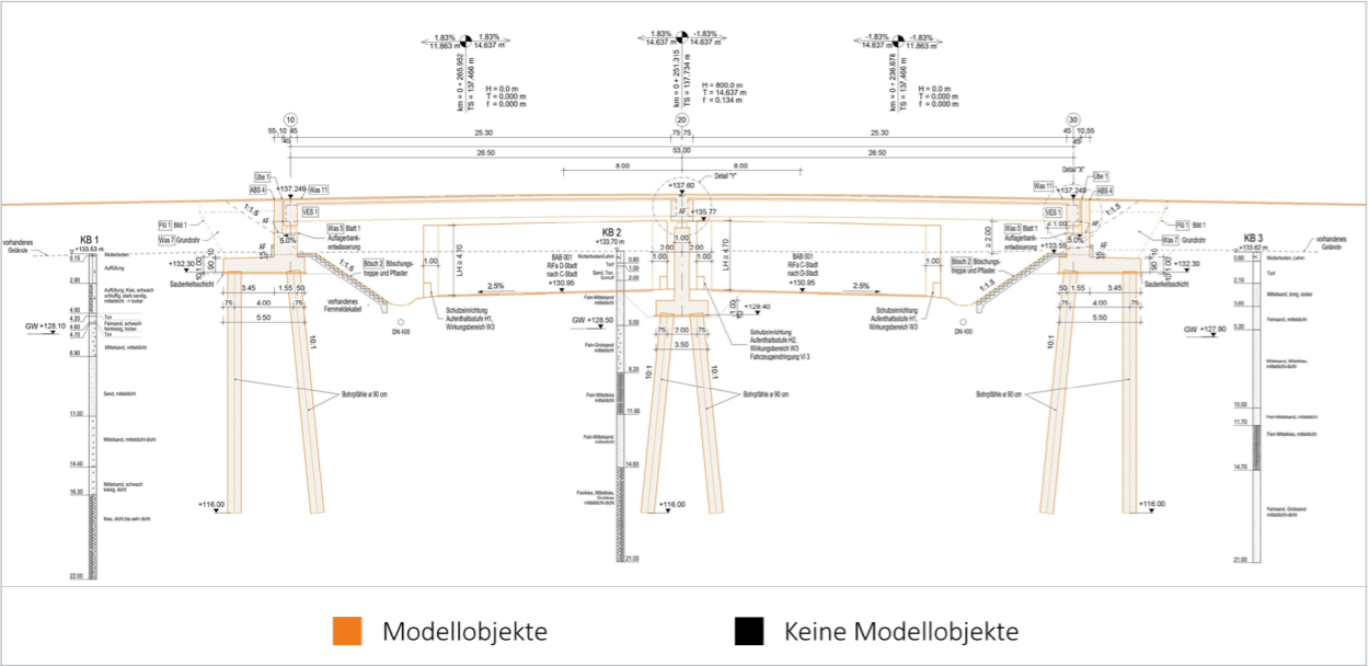
Abbildung 8: Gegenüberstellung von aus dem Modell abgeleiteten und manuell ergänzten Objekten einer exemplarischen Plandarstellung (© Schüler-Plan)
